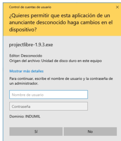
Ilustración 1 Pantallazo projectlibre-1.9.3.exe
